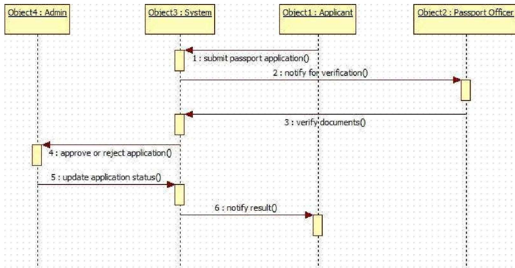
Fig 5.6 Simple sequence diagram PAS
