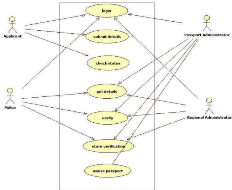
Fig 5.4 Simple Use case diagram PAS
