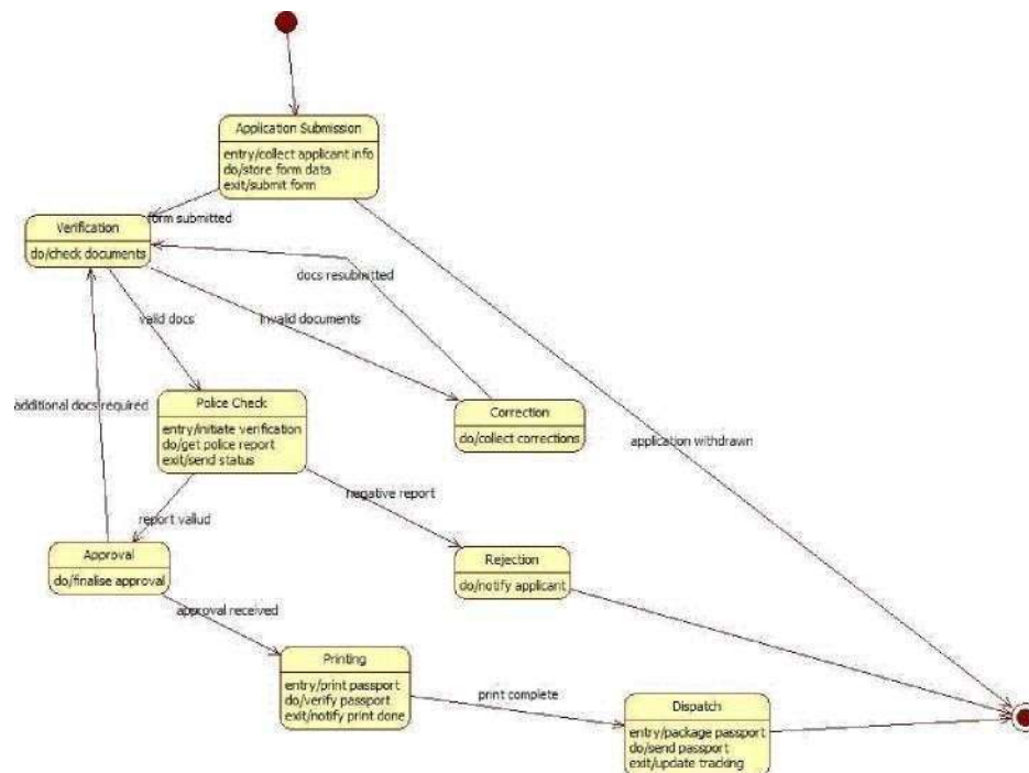
Fig 5.2 Simple state diagram PAS
